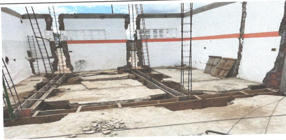
MONTAGEM DE FORMAS DE VIGAS BALDRAME
